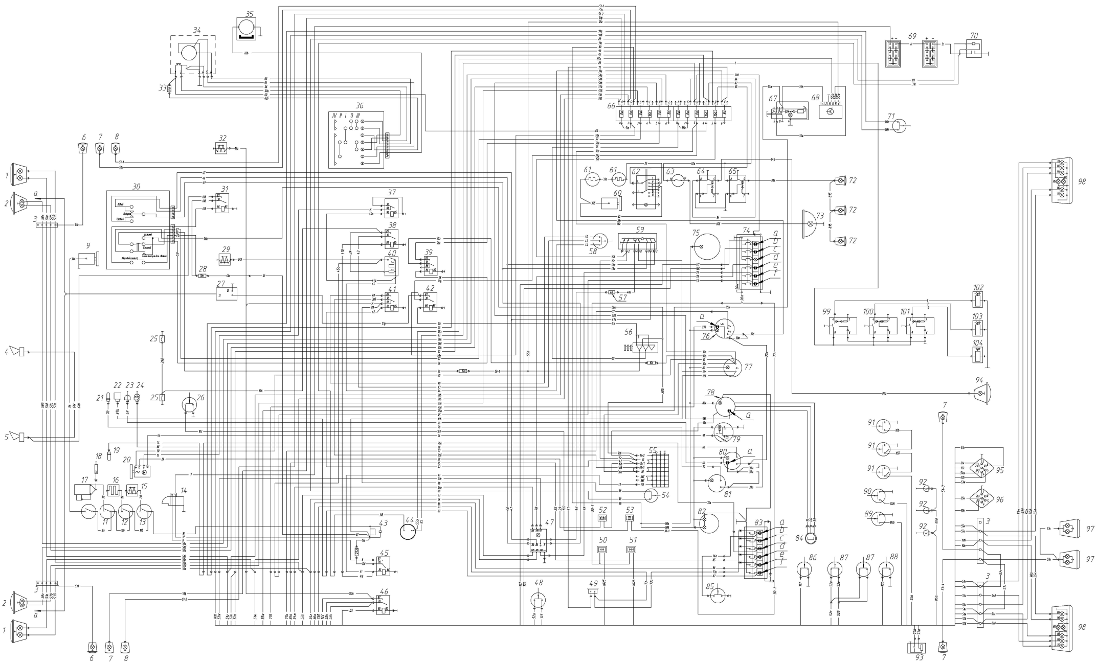
Рис. 59. Схема электрооборудования (НХ)
