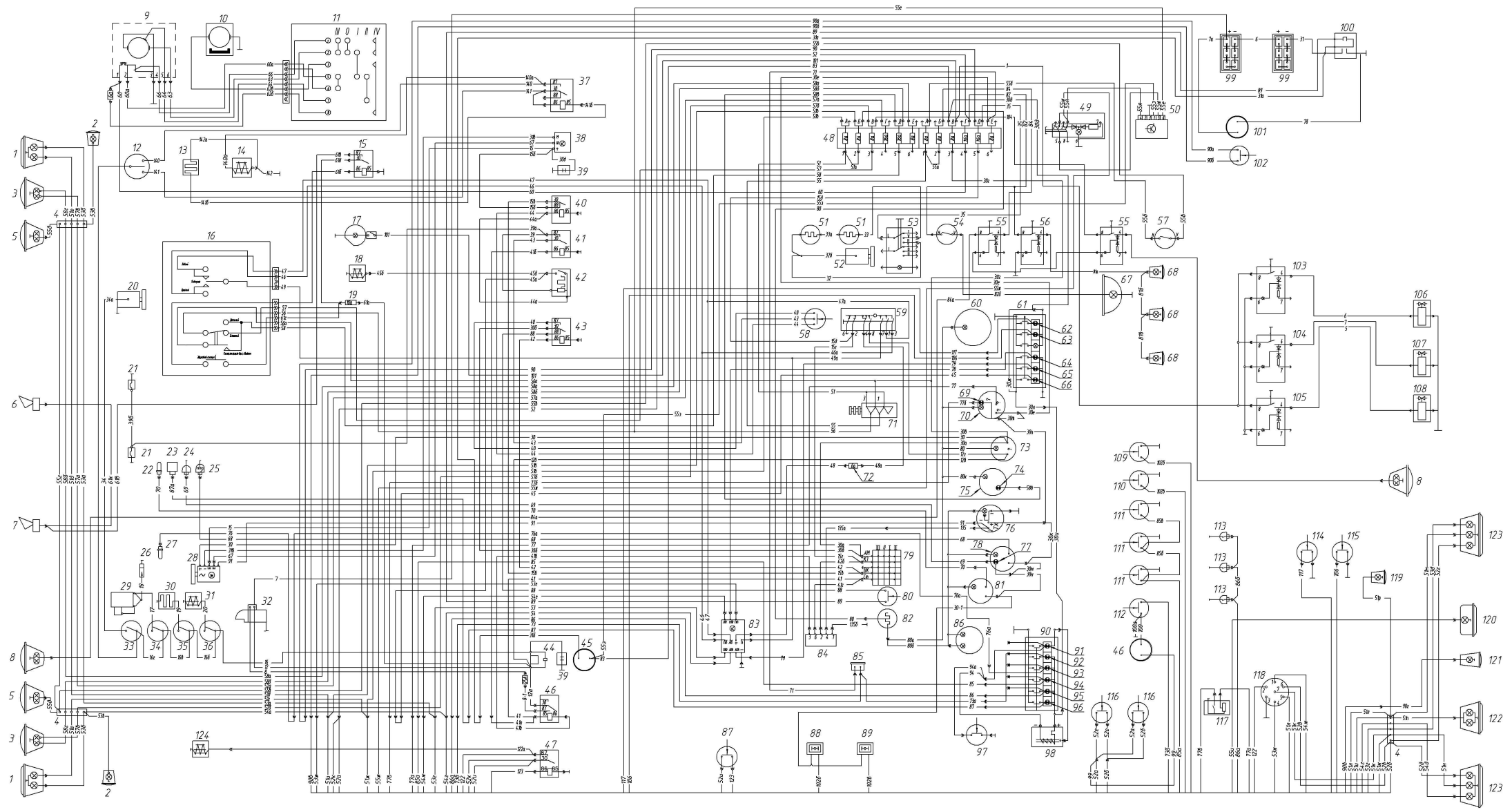
Рис. 21. Схема электрооборудования (МО)
