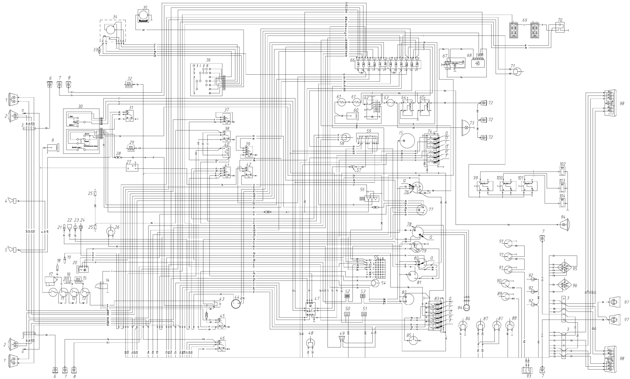
Рис. 32. Схема электрооборудования автомобилей Урал-4320-41, Урал-4320-40
