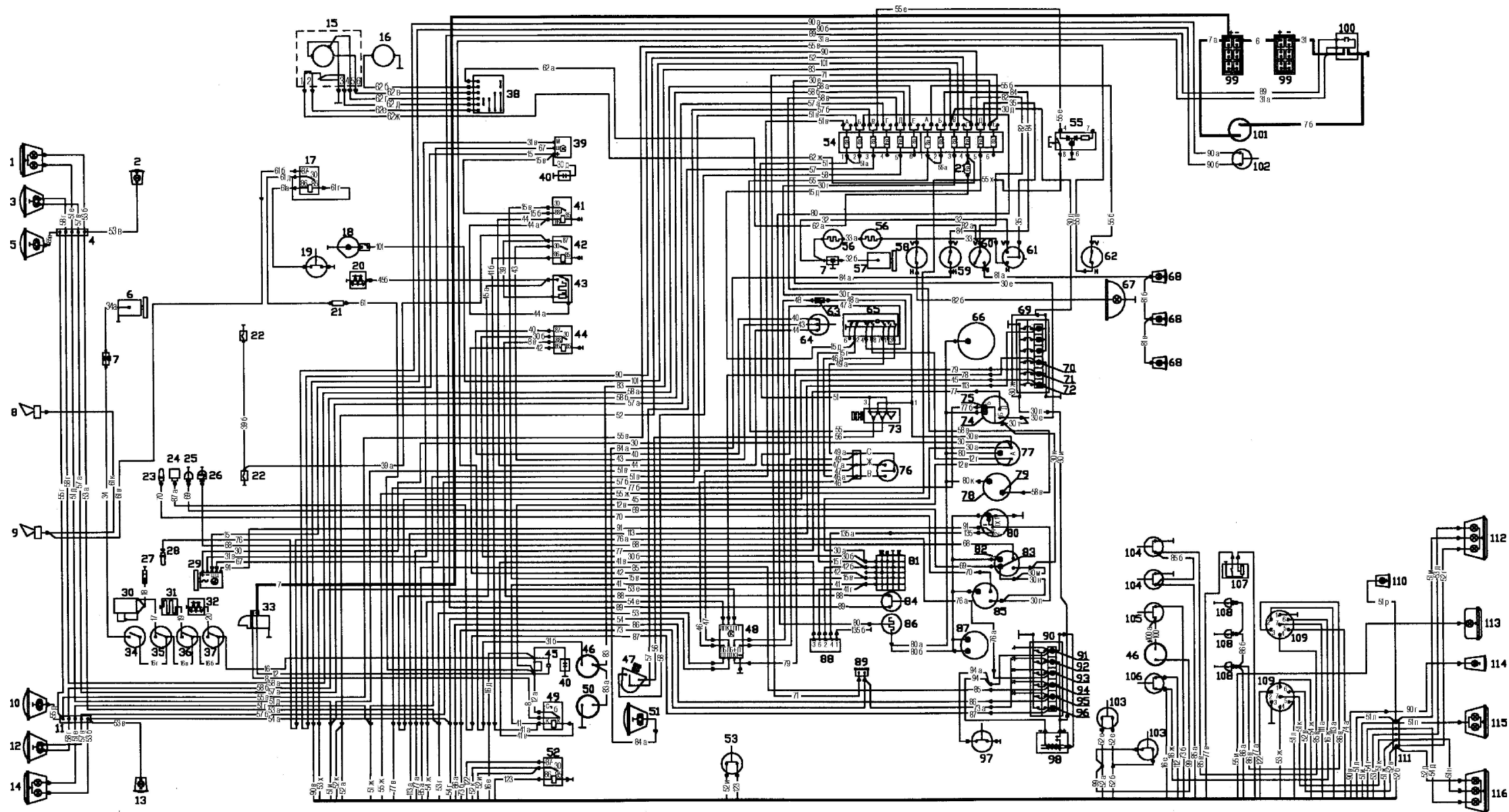
Рис. 86. Схема электрооборудования автомобилей Урал-4320-10, Урал-4320-31 (исполнение МО)
