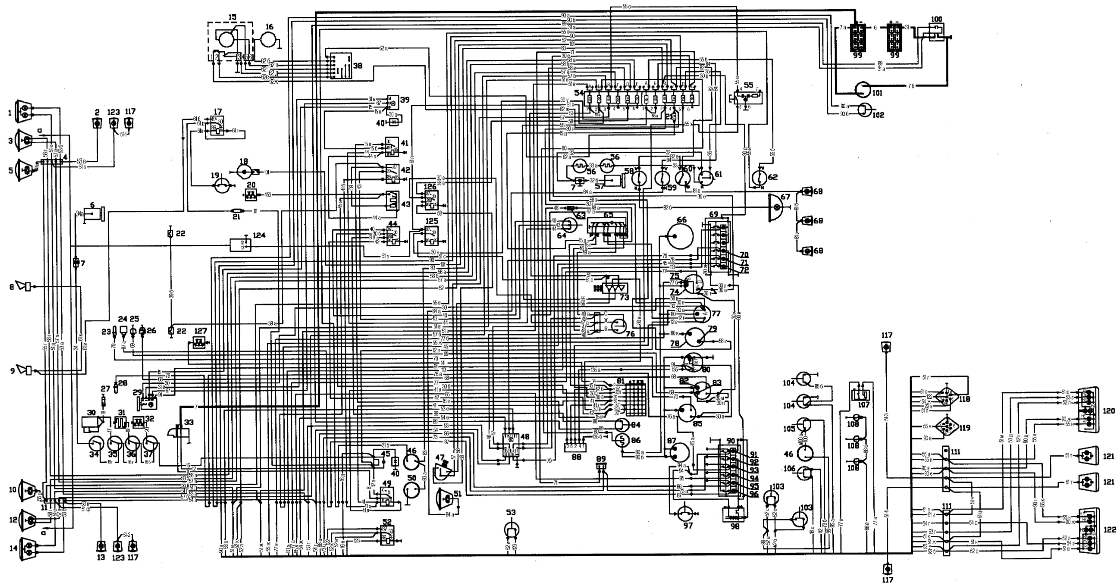
Рис. 86. Схема электрооборудования автомобилей Урал-4320-10, Урал-4320-31 (исполнение НХ)
